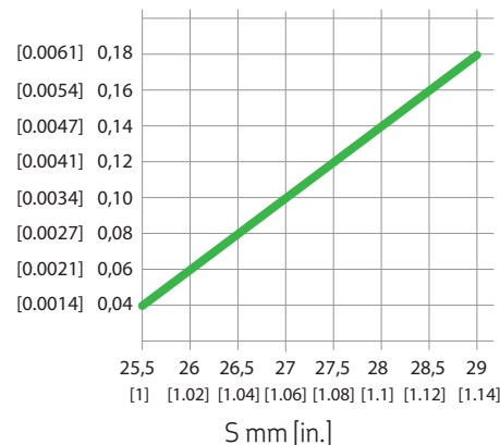
Ajuste del caudal en el elemento de bomba R Fig. 10
