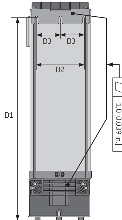
Taladros de montaje para bombas con depósitos de 11 l [2.9 gal.] ó 15 l [3.96 gal.] Fig. 7
