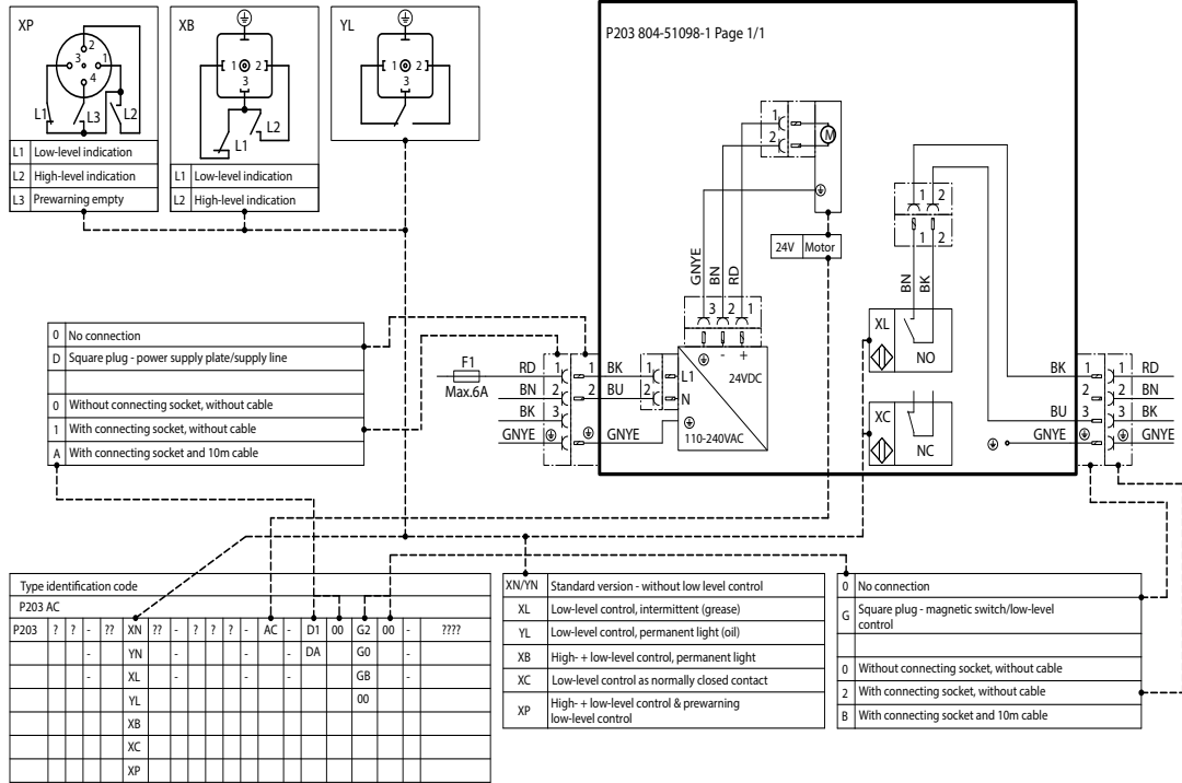
Esquema de conexiones P203 V AC sin pletina de mando Fig. 32
