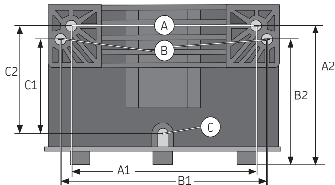
Puntos de fijación en la carcasa de la bomba de la bomba P203 Fig. 6
