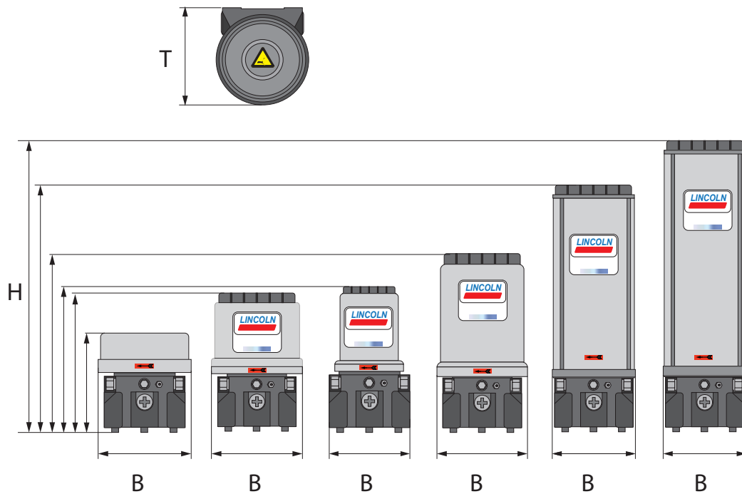
Medidas de instalación mínimas Fig. 5
