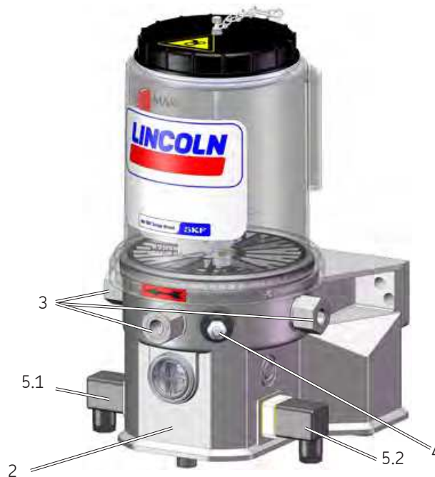
Resumen, descripción de la función de bombas sin placa seguidora Fig. 2
